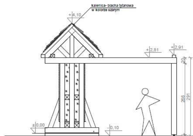
ELEWACJA POŁUDNIOWA
