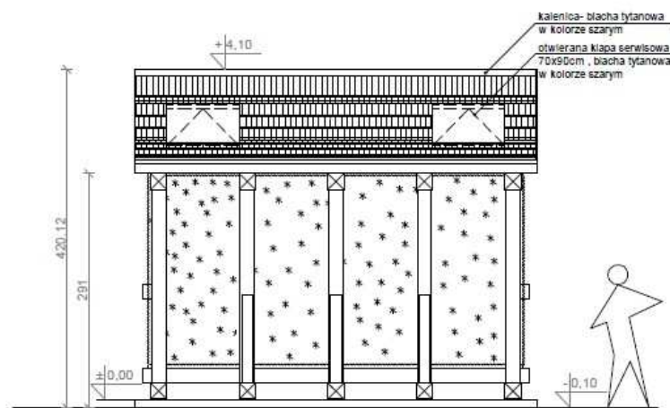
ELEWACJA ZACHODNIA FRONTOWA
